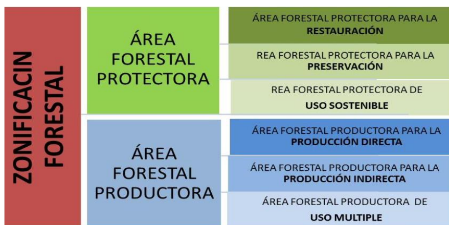
Figura 23. Zonificación forestal de las unidades administrativas de ordenación forestal, Plan General de Ordenación Forestal del departamento del Chocó (tomado de Codechocó, 2019).
