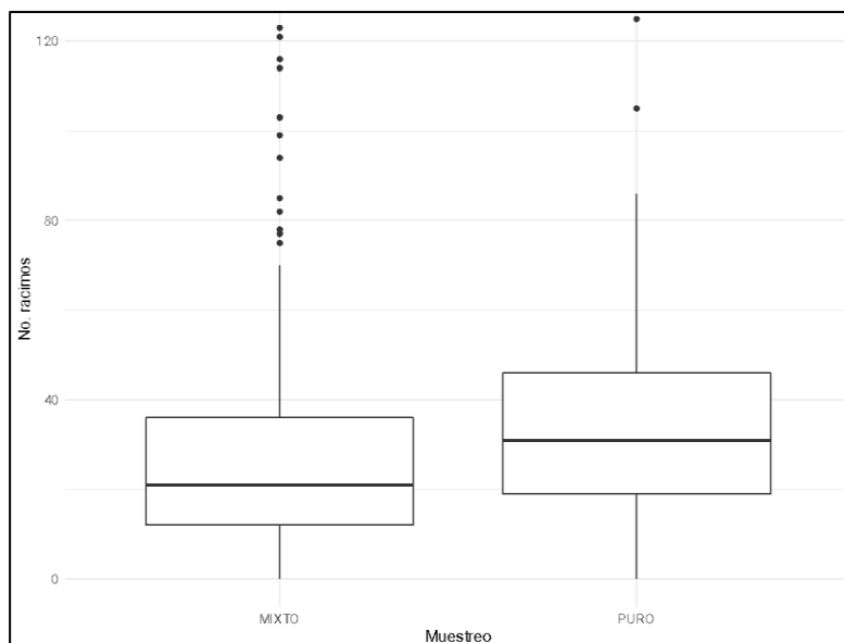
Figura 20. Cantidad de racimos producidos por macolla en naidizal mixto y naidizal puro. Existe diferencia significativa entre la producción de racimos entre naidizal mixto y puro (Kruskall-Wallis, p < 0,05^* ).
